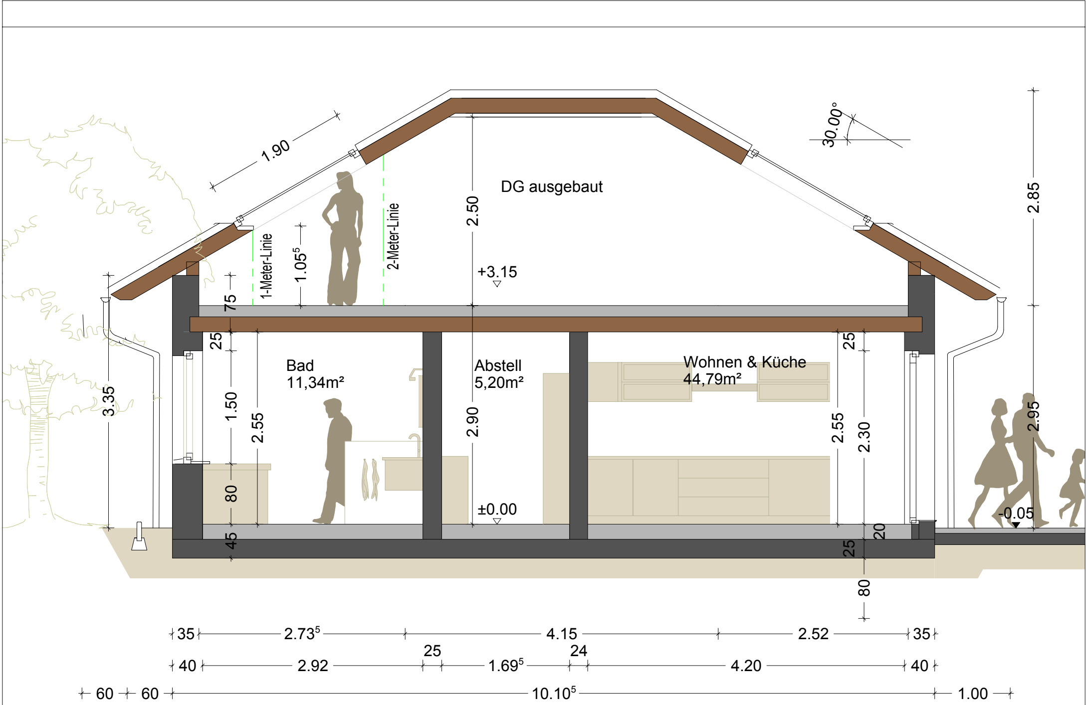
Schnitt bei ausbaufähigem DG 1 : 50 24.10.2014
